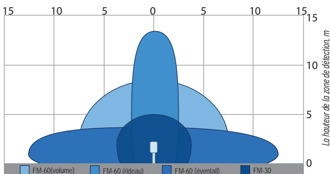
La zone de détection du détecteur FM-60 (rideau)
